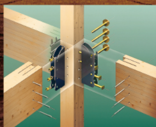
MJ(メタルジョイント)接合
