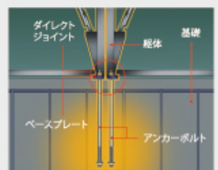
建物にかかった力を、効率良く地面に逃がす 「ダイレクトジョイント」
